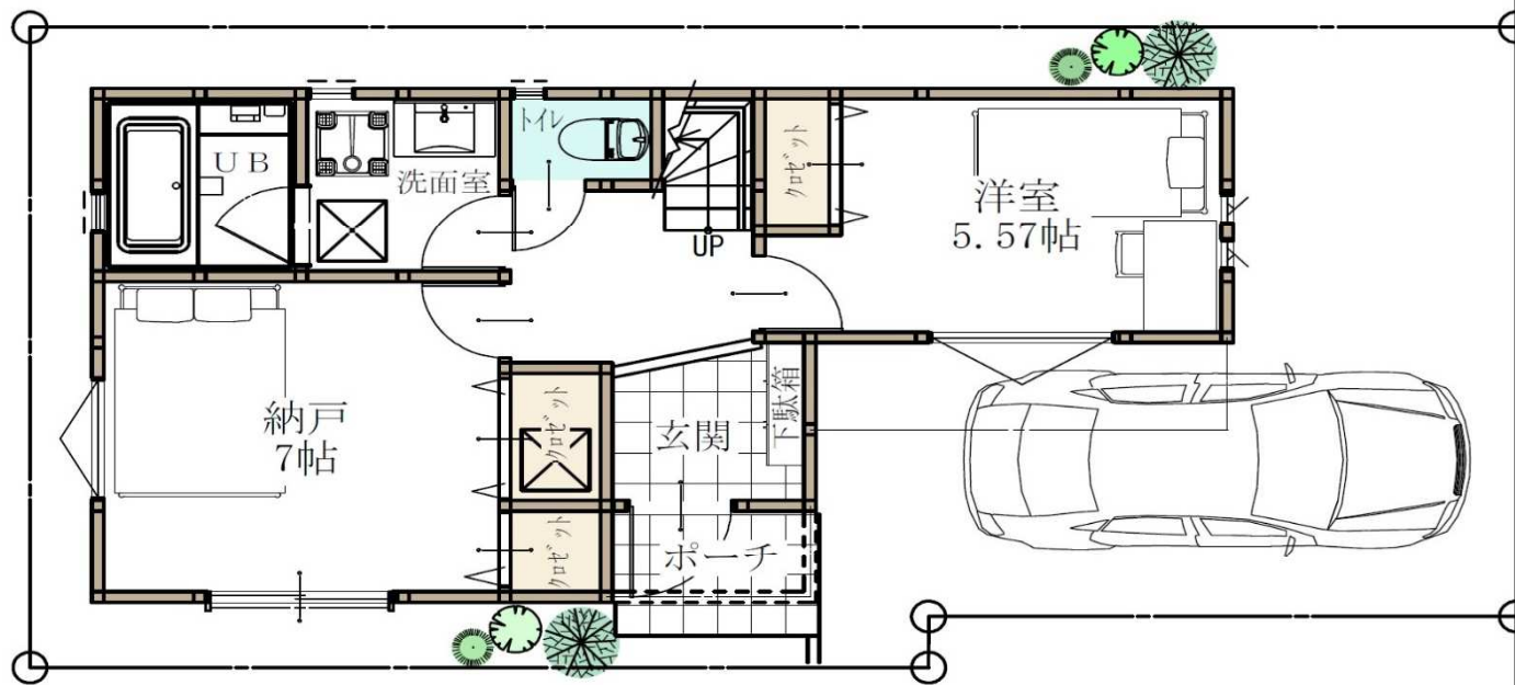
1階 平面図
